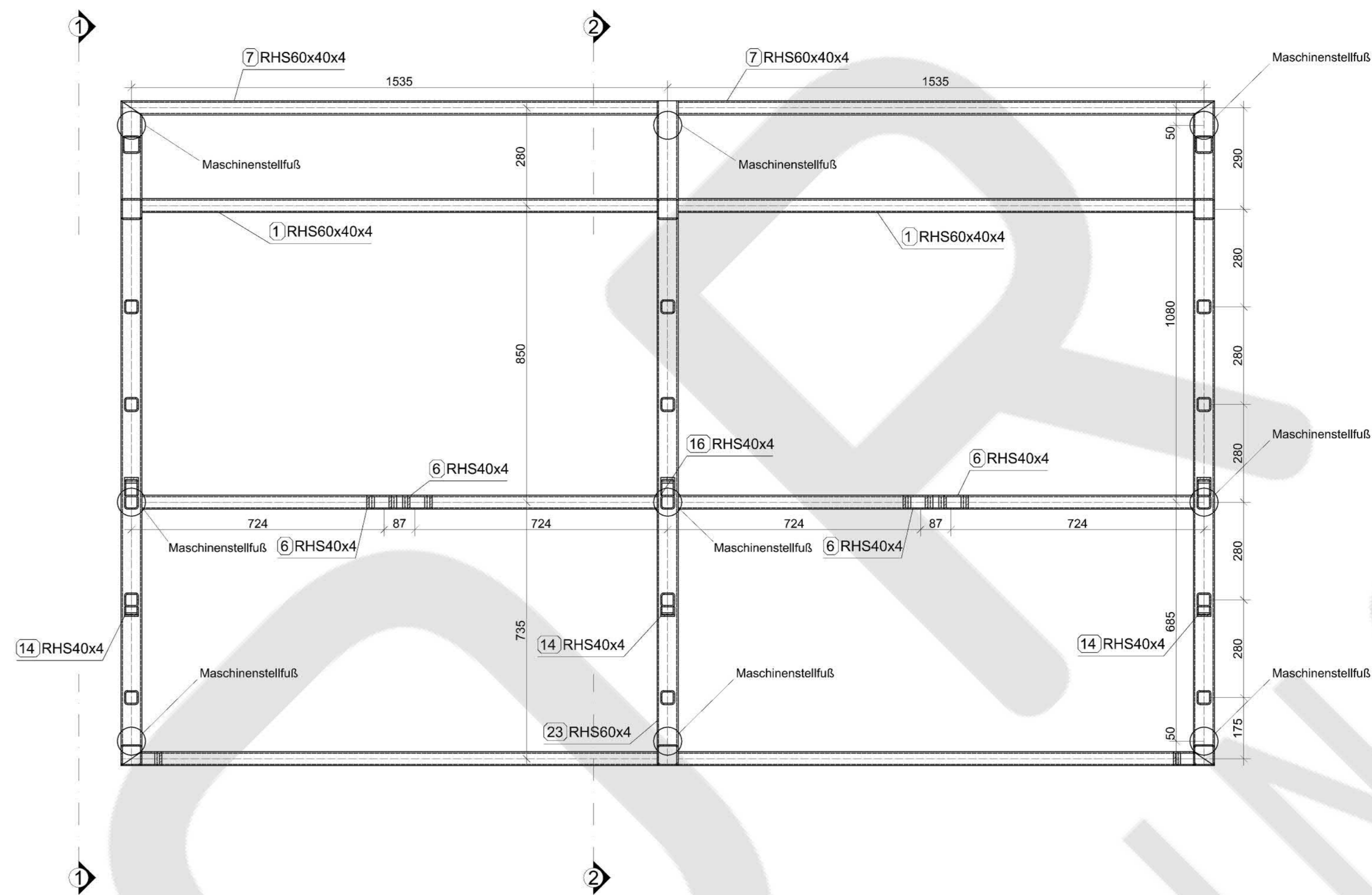
Schnitt 2-2
