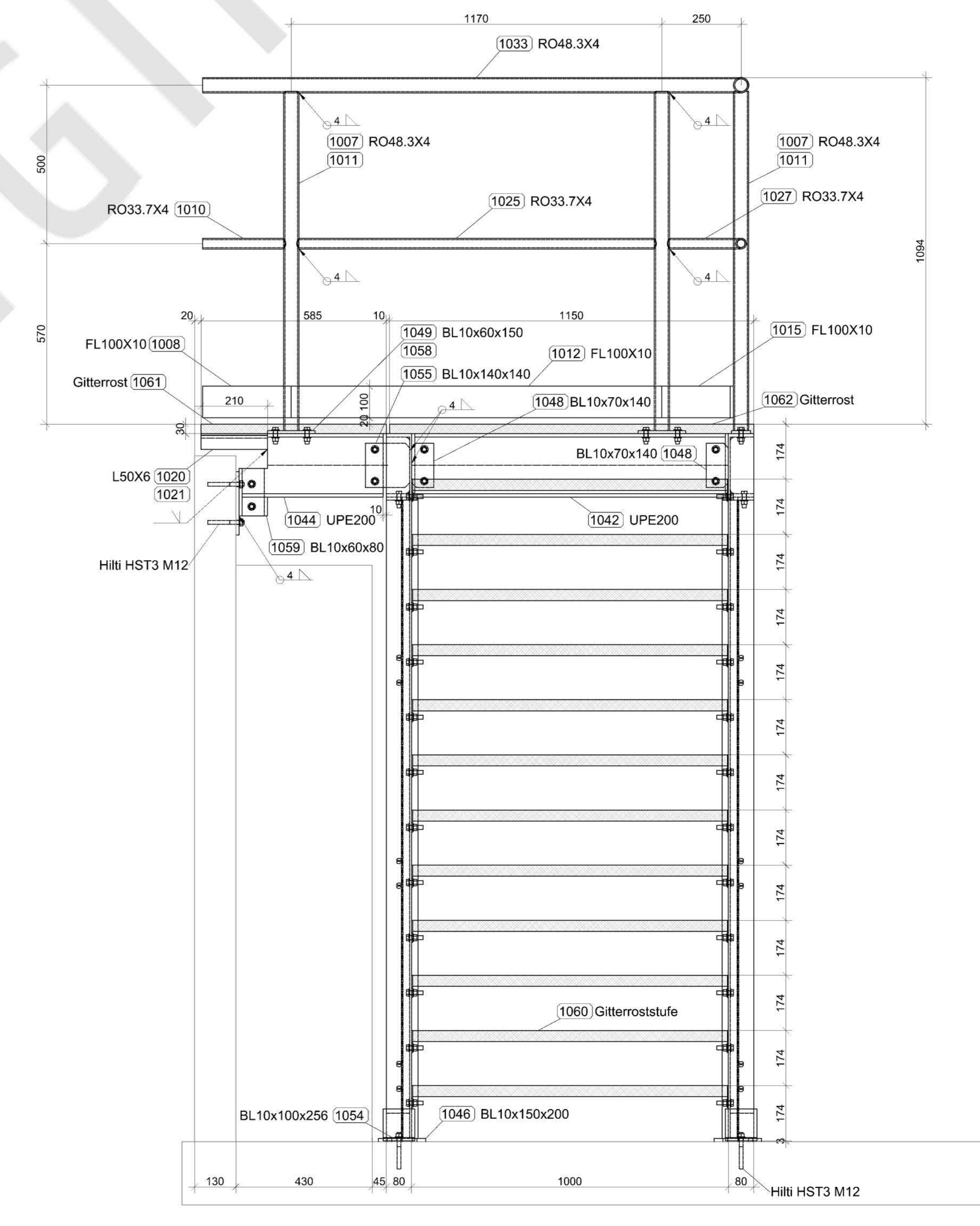
Schnitt 2-2
